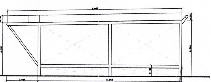
รูปด้าน D ขนาดจริง 1:10
