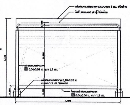
รูปด้าน A ขนาดตัว 1:10
