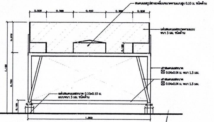
รูปด้าน C ขนาดตัว 1:10
