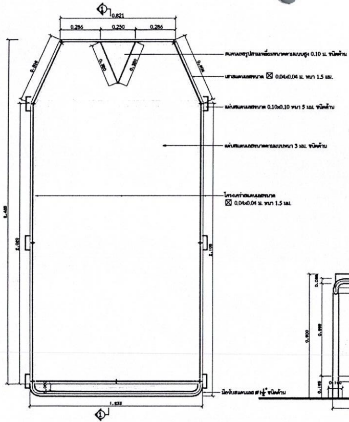
แปลนขยายโตะและต้นเลดคัตเลือกส้วน้ำ (ขนาดกลาง) ขนาดจริง 1:50
