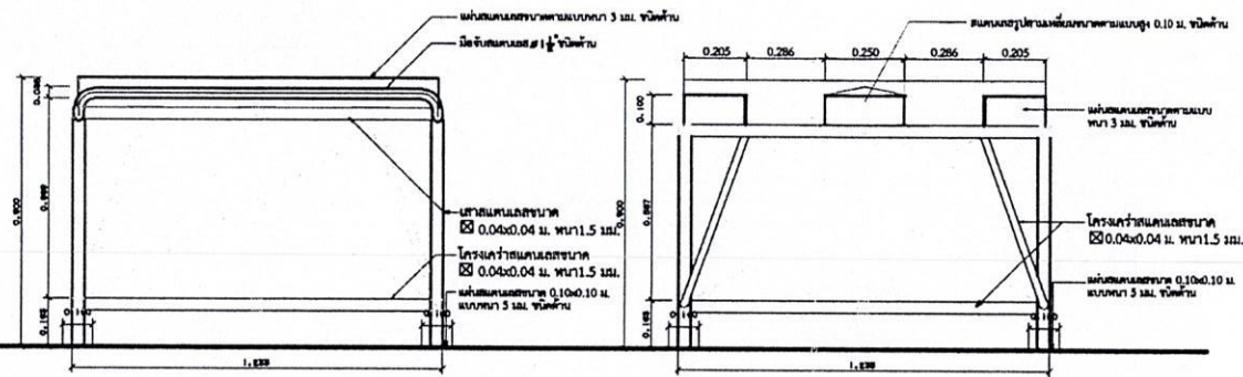
รูปด้าน A ขนาดจริง 1:10
